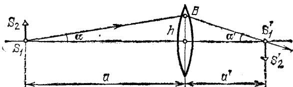
Рис. 212. Угловое увеличение линзы \gamma = \tan \alpha' / \tan \alpha = a/a'
