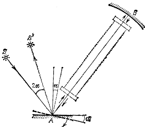
Рис. 308. К определению скорости света по методу вращающегося зеркала
