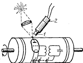
Рис. 146. Схема передающего устройства фототелеграфа:
