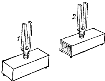
Рис. 40. Резонанс камертонов
