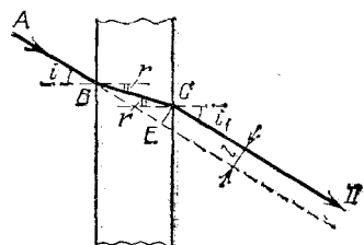
Рис. 188. Преломление в плоскопараллельной пластинке
