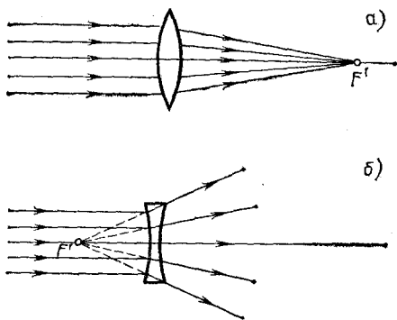
Рис. 199. Действительный фокус собирающей линзы ( a ) и мнимый фокус рассеивающей линзы ( b )
