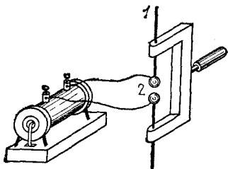
Рис. 122. Схема вибратора Герца
