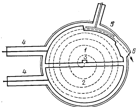
Рис. 392. Схема камеры циклотрона: 1, 2 — дуанты. Дуанты представляют собой нечто вроде половинок очень плоской консервной банки, разрезанной по диаметру; 3 — источник ионов, 4 — входы переменного напряжения на дуанты, 5 — пластина, заряженная отрицательно и служащая для отклонения ускоренных ионов в окно 6, через которое ускоренный пучок выводится наружу. Штриховая спираль — траектория иона
