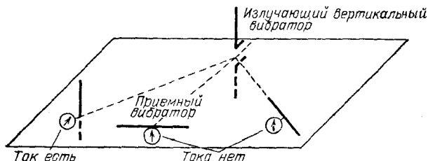
Рис. 133. Наиболее сильный ток в индикаторе возникает только при вертикальном расположении приемного вибратора. При любом горизонтальном положении вибратора тока нет
