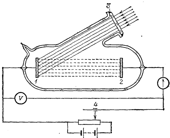
Рис. 331. Схема опыта по измерению фототока и скорости фотоэлектронов: 1 — освещаемая пластина (катод), 2 — вспомогательный электрод (анод), 3 — окошко, прозрачное для ультрафиолетового излучения, 4 — движок потенциометра
