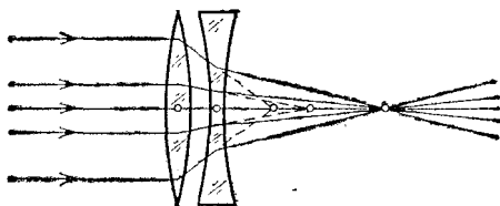
Рис. 232. Исправление сферической аберрации путем комбинирования собирающей и рассеивающей линз
