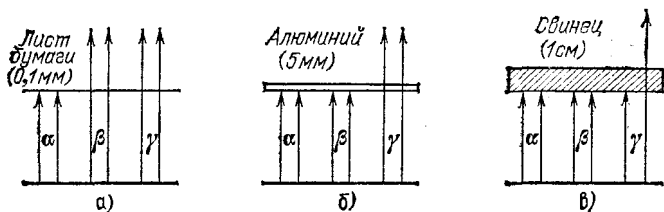
Рис. 378. Поглощение радиоактивных излучений веществом
