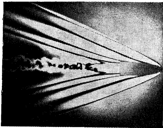
Рис. 294. Изображение ударных волн, создаваемых летящей пулей лящей пули, полученное с помощью двухэкспозиционной голограммы. Видны интерференционные полосы в области ударной волны.
