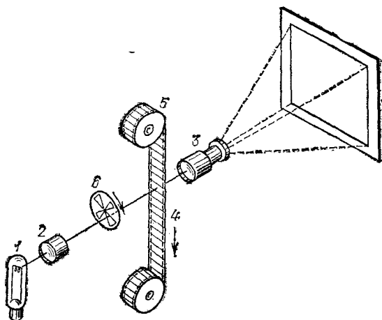
Рис. 241. Схема простейшего киноаппарата: 1 — источник света; 2 — конденсор; 3 — проекционный объектив; 4 — фильм; 5 — лентопритяжный механизм; 6 — obturator
